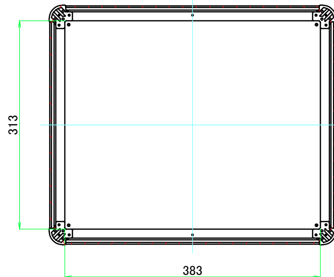
C-C ( 1 : 5.5 )
