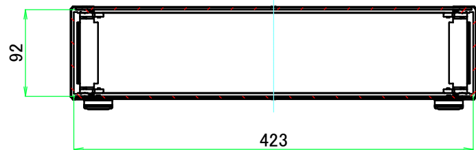
A-A ( 1 : 5.5 )
